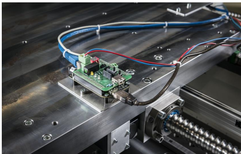
Kleiner Stecker, große Wirkung: Der Plug-and-Play-Adapter überwindet Sprachbarrieren zwischen Maschinen und macht das Umrüsten von Anlagen leichter. (Bild: KIT)
