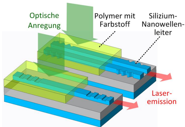
Organischer Laser auf einem Silizium-Photonik-Chip: Eine optische Anregung von oben führt zu Laserlicht im Wellenleiter. (Bild: KIT)
