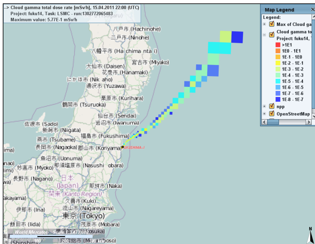
Abbildung 1: Fahngammastrahlung (Bildschirmausdruck RODOS), Fall mittlere Abschätzung mit Startzeitpunkt der Freisetzung am 15.04.2011, 12:00 UTC (Lesehilfe: 1E-3 bedeutet 1 \times 10^{-3} oder 0,001)
