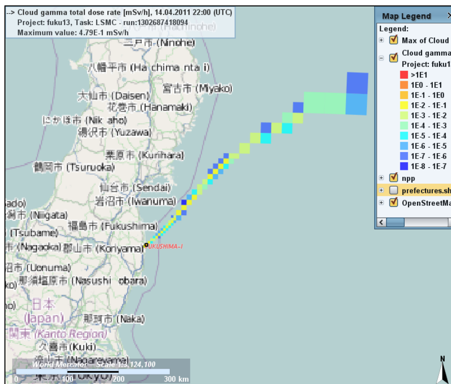
Abbildung 1: Fahngammastrahlung (Bildschirmausdruck RODOS), Fall mittlere Abschätzung mit Startzeitpunkt der Freisetzung am 14.04.2011, 12:00 UTC (Lesehilfe: 1E-3 bedeutet 1 \times 10^{-3} oder 0,001)
